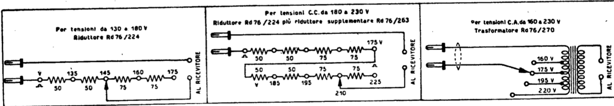
MARELLI - Mod. 9U65/E - Gamme: OL da 145 a 310 kc; OM da 514 a 1570 kc; OC1 da 5,5 a 9,7 Mc; OC2 da 9,4 a 16,5 Mc. MF a 470 kc. Altop. come 9U65 C. Tensioni placche e schermi 96 V, catodo finale 6,4 V.
